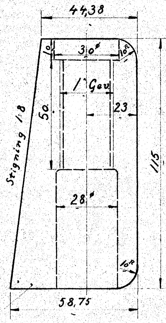
3. Kobbeltang m /og 2 - 3 og 4 Hjul
