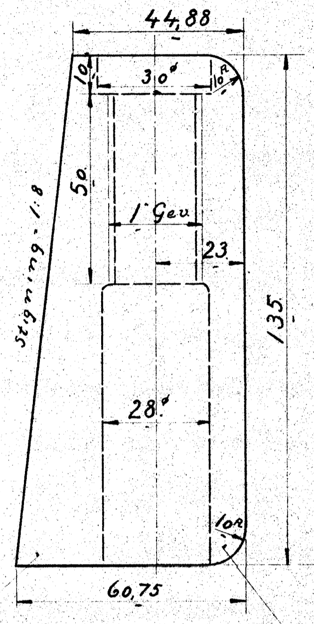
2. Kobbeltang m /2 og 3 Hjul.
