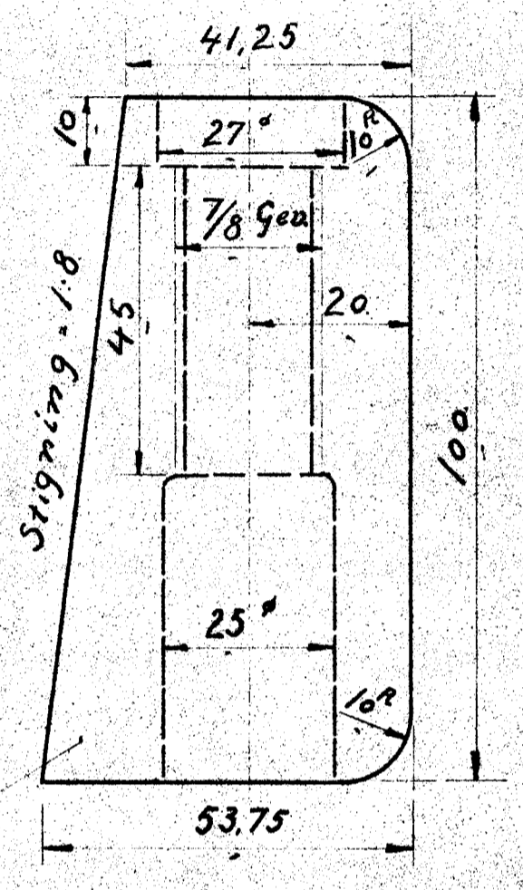
3. Kobbeltang m /og 2 - 3 og 4 Hjul
